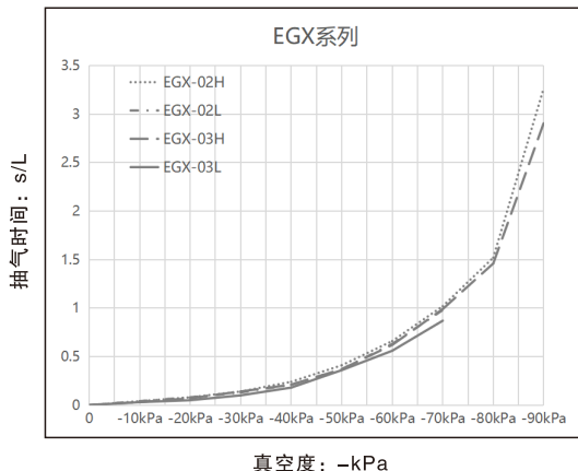
EGX 不同真空度 (-kPa)的抽气时间(s/L)
