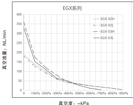
EGX 不同真空度 (-kPa)的真空流量(NL/min)
