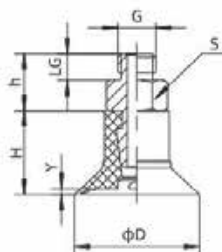
SZF15□-M5M 外螺纹连接
