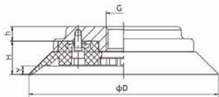
SZF75-150 内螺纹连接
