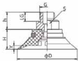
SZF40-50 外螺纹连接
