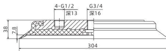
SZF300 内螺纹连接
