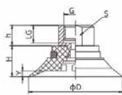
SZF40-50 内螺纹连接
