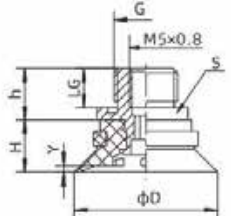
SZF20-30 外螺纹连接
