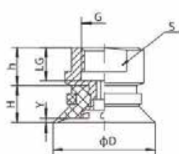
SZF20-30 内螺纹连接
