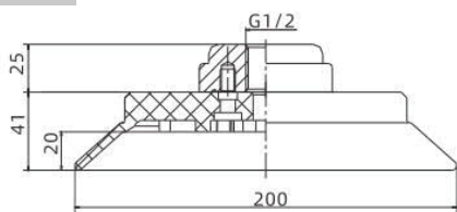
SZF200 内螺纹连接
