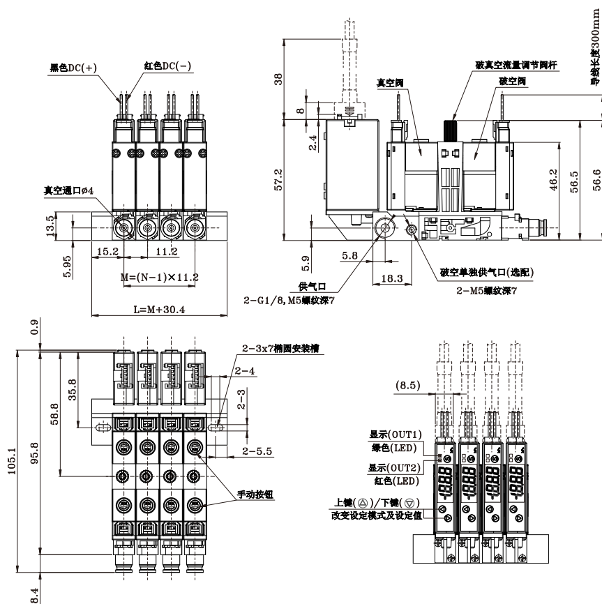
EZBZ□-N/P帶真空压力表
