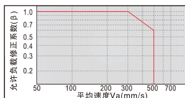
图三：允许负载修正系数（ \beta ）
