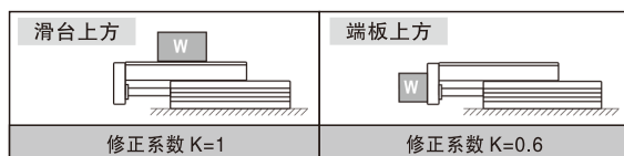
图二：治具安装方式修正系数（K）
