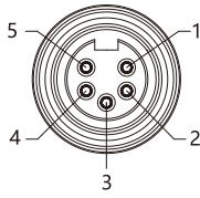
电源输出接口（7/8” 孔端，Female）
