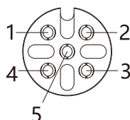
IO-Link接口（8XM12, A编码,Female）
