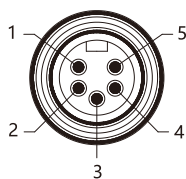
电源输入接口（7/8” 针端，Male）
