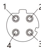
总线接口（2XM12, D编码,Female）
