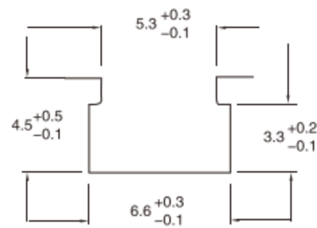
HX-65系列沟槽尺寸图*
