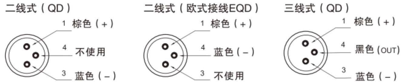
M8/M12公头接线图
